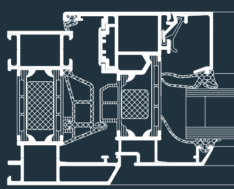
Schüco Fenster AWS 70 RL.HI Maßstab 1:2 Schüco Window AWS 70 RL.HI Scale 1:2
