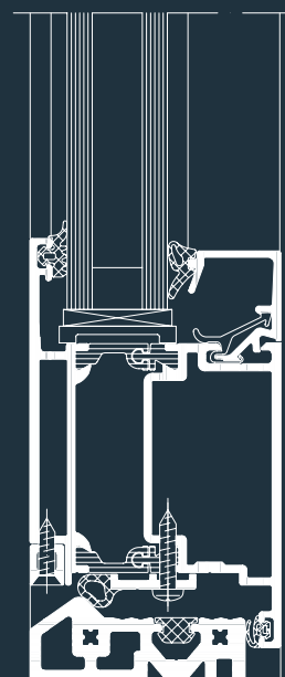
Schüco Tür ADS 60, Maßstab 1:2 Schüco Door ADS 60, Scale 1:2
