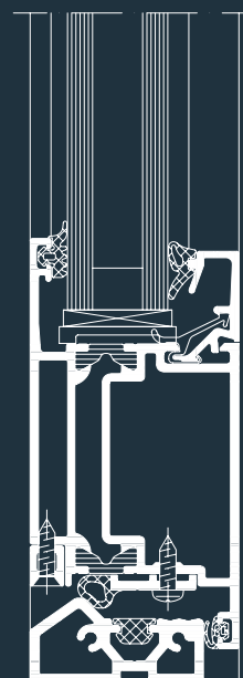
Schüco Tür ADS 50.NI, Maßstab 1:2 Schüco Door ADS 50.NI, Scale 1:2
